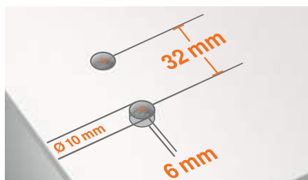
Montering utan grytborrning
