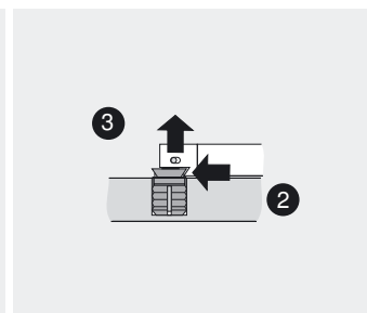
Främre demontering
