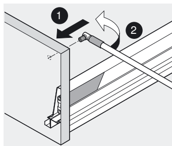
Främre montering
