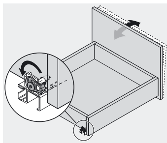
560/566: lutning över skena
