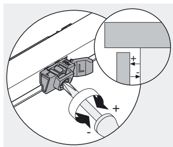
Djupjustering – TIP-ON 56X/550/551
